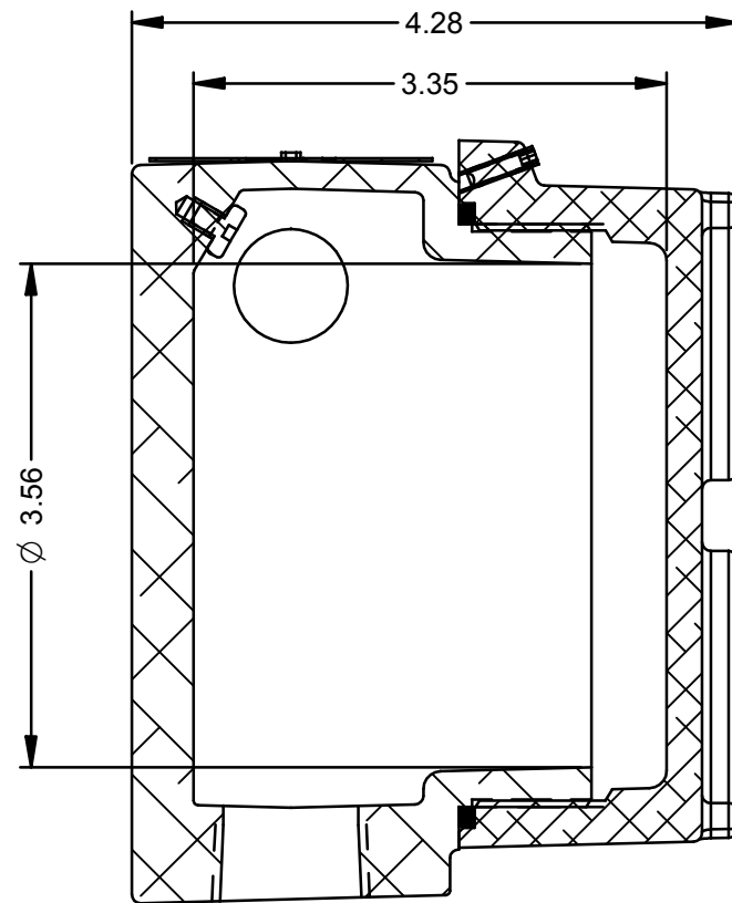
SECTION A-A 1:1.5
