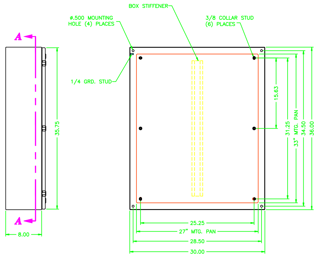
SECTION A-A
